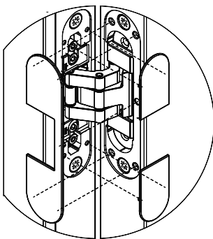
30/24×120
